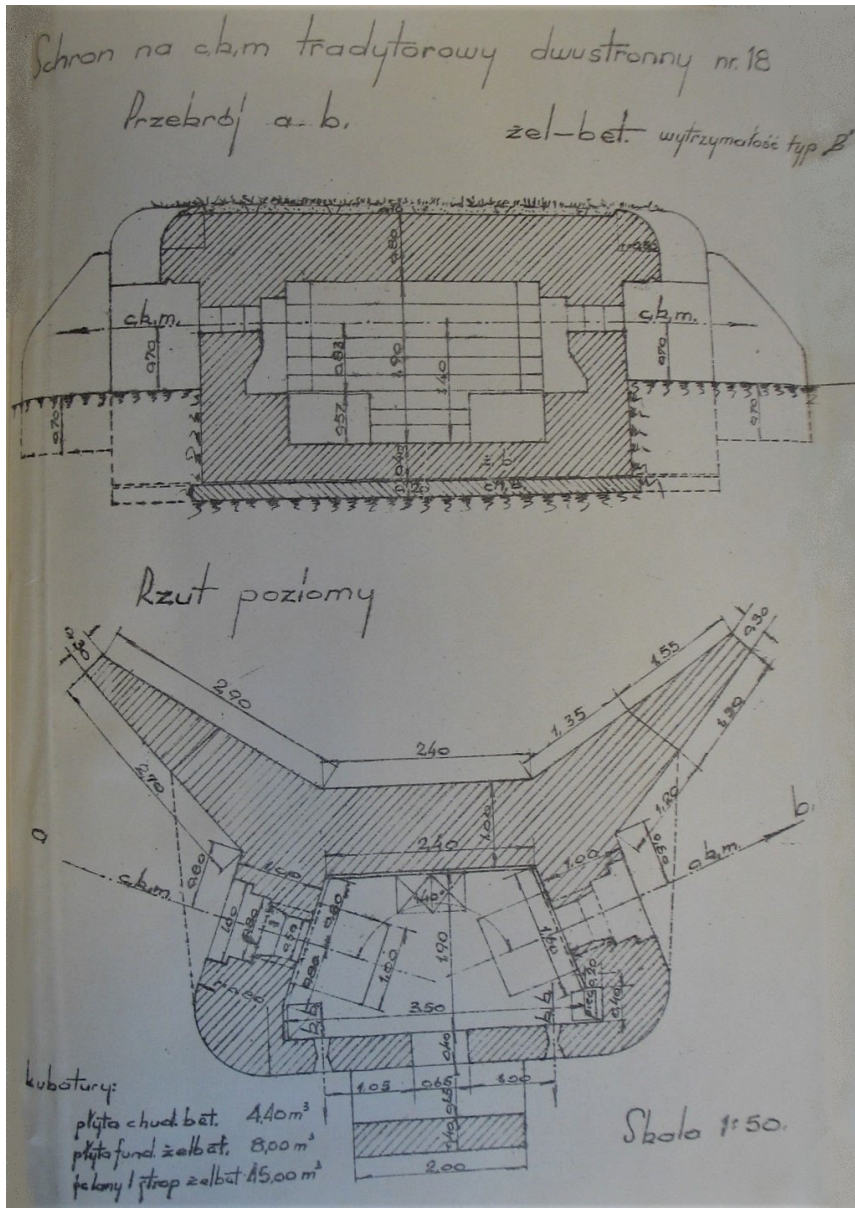
Projekt budowy dwustrzelnicowego schronu bojowego o cofniętych kątach Źródło: Instrukcja Saperska. Umocnienia polowe, cz. III (projekt), z. II, Schrony żelbetowe i betonowe, Sztab Główny Inspektorat Saperów 1939
